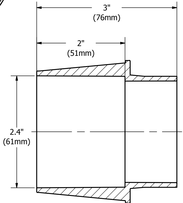
SECTION A-A
